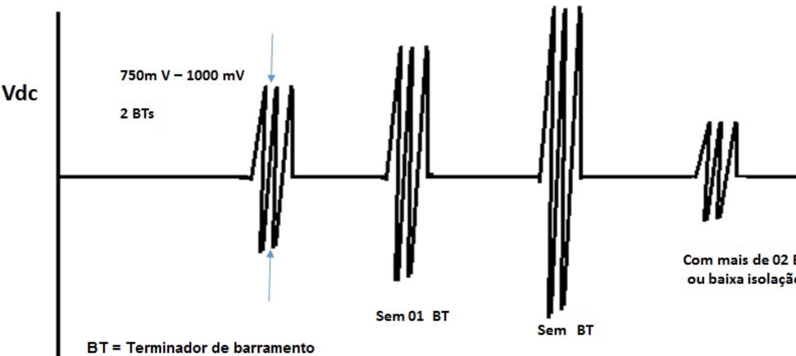
Figura 12 – Formas de onda típicas do Profibus-PA, de acordo com a terminação.
