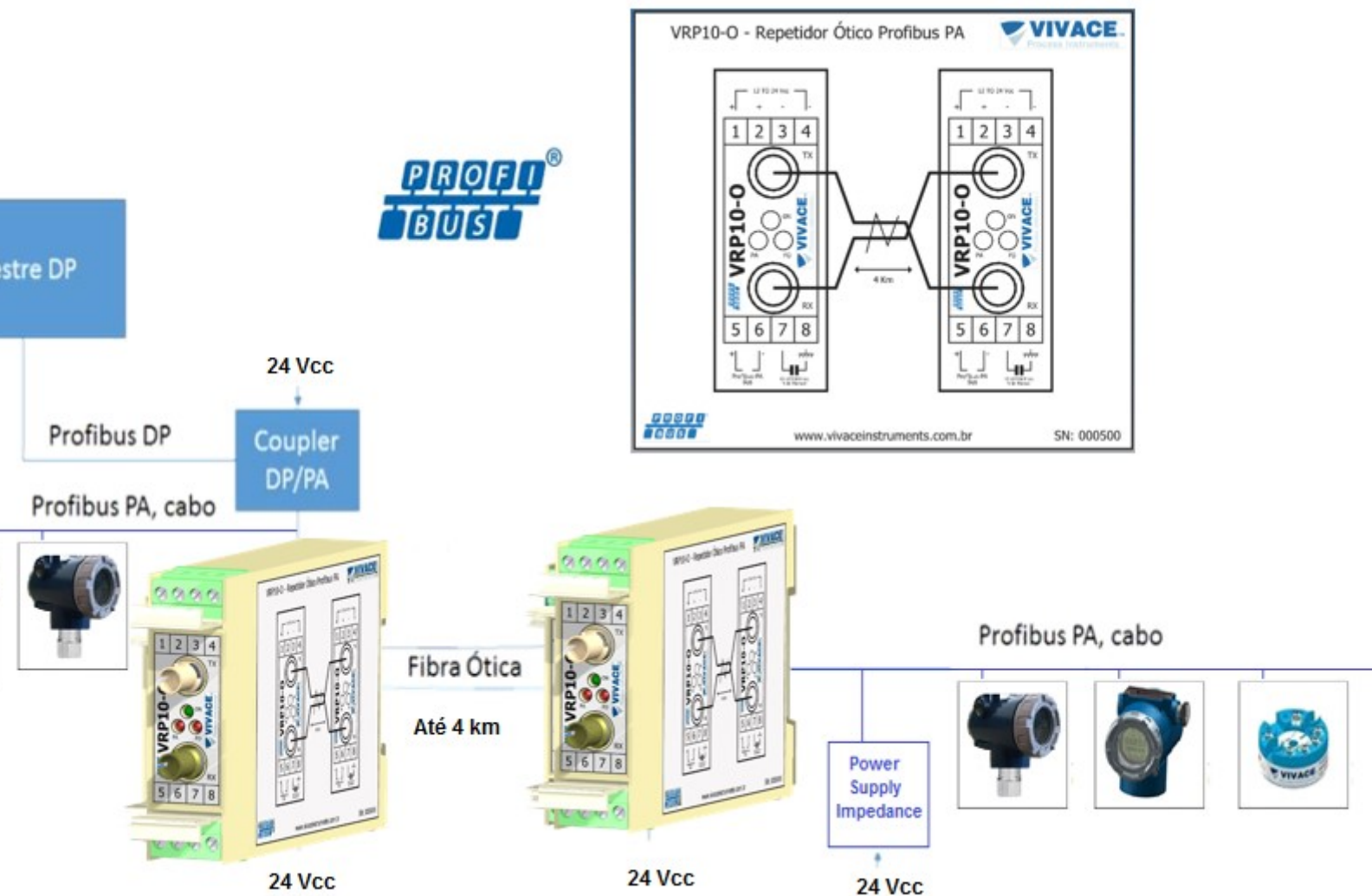
Figura 16– Aplicação típica do VRP10-O, expandindo a rede Profibus-PA.
