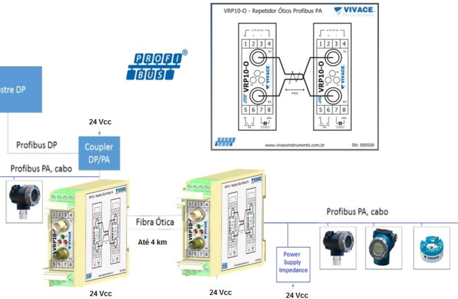
Figura 16– Aplicação típica do VRP10-O, expandindo a rede Profibus-PA.
