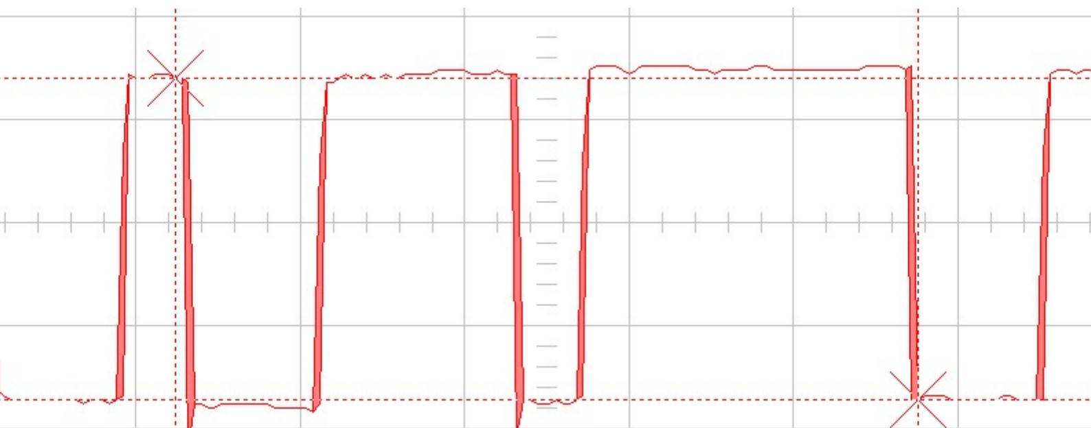
Figura 8 – Sinal corrigido após a instalação do repetidor DP.
