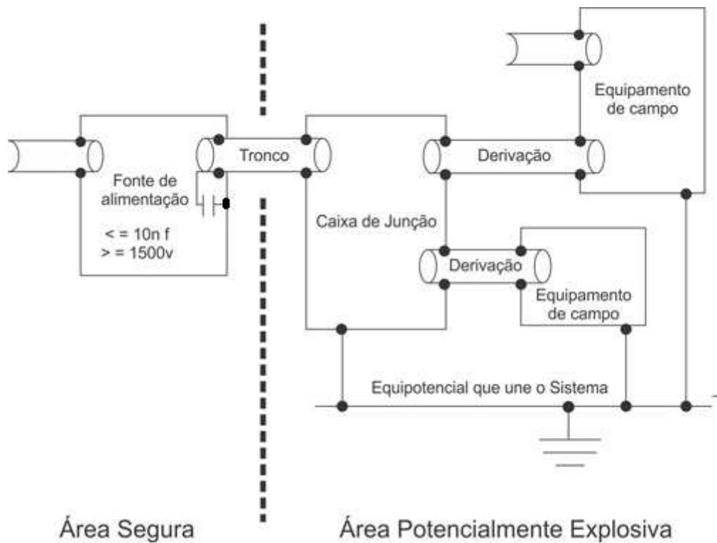
Figura 15 – Aterramento capacitivo.
