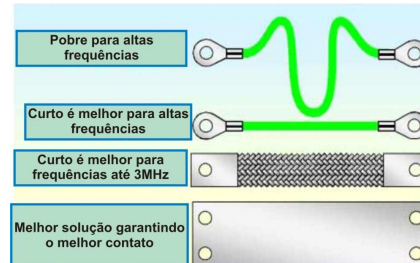
Figura 4 – Material para Equipotencializar.
