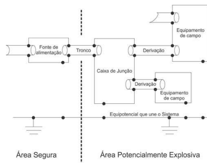
Figura 14 – Combinação Ideal de shield e aterramento.
