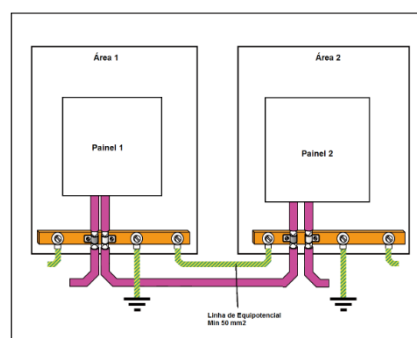
Figura 16 – Linha de Equipotencial.
