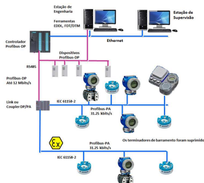
Figura 1 – Arquitetura típica Profibus.
