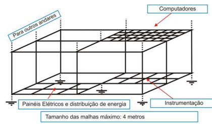
Figura 2 – Equipotencialização.
