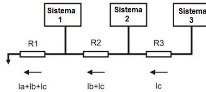
Figura 7 – Aterramento em multipontos inadequado
