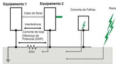
Figura 8 – Aterramento ao nível dos equipamentos na prática
