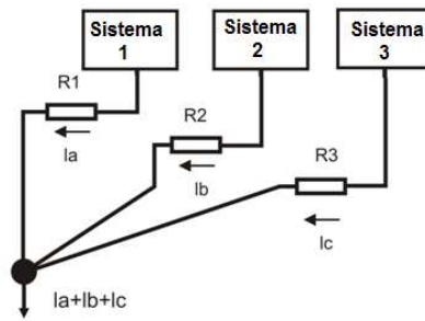
Figura 6 – Aterramento adequado, em um único ponto.
