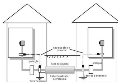
Figura 18 – Detalhe de cabeamento em áreas distintas com potenciais de terras equalizados.
