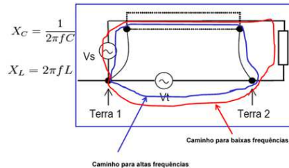
Figura 12- Efeito blindagem x aterramento em dois pontos.
