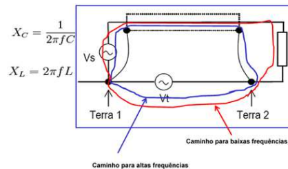
Figura 12- Efeito blindagem x aterramento em dois pontos.
