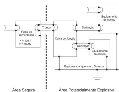
Figura 15 – Aterramento capacitivo.
