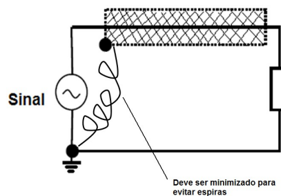
Figura 13- Deve-se minimizar o comprimento da ligação blindagem-referência pois funciona como uma bobina.
