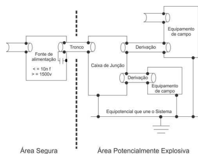
Figura 15 – Aterramento capacitivo.
