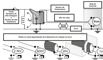
Figura 5 – Exemplo da importância do aterramento e equipotencialização e sua influência no sinal.
